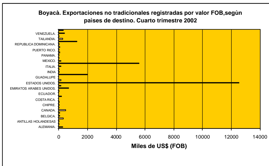
Grafico 4
