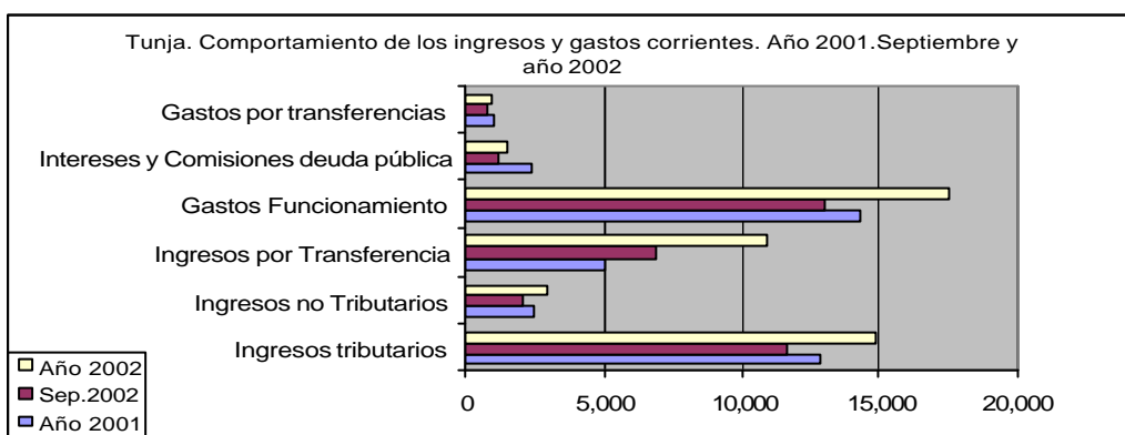
Grafico 8
