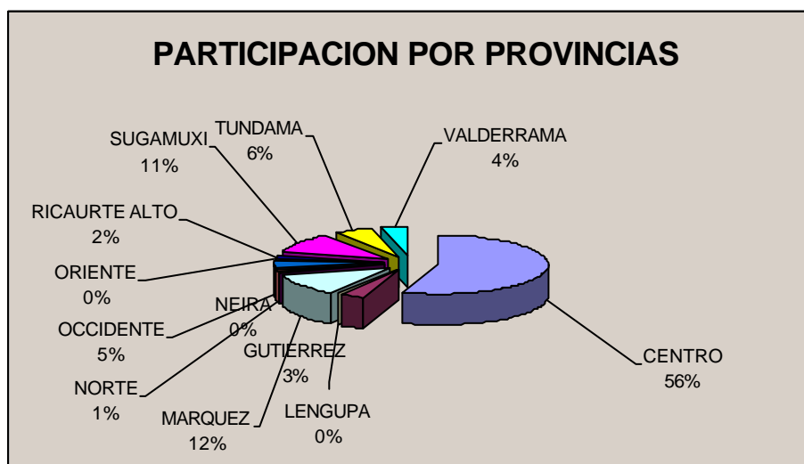
Gráfico No1
