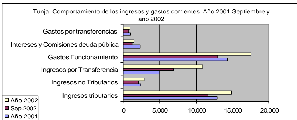
Gráfico 9
