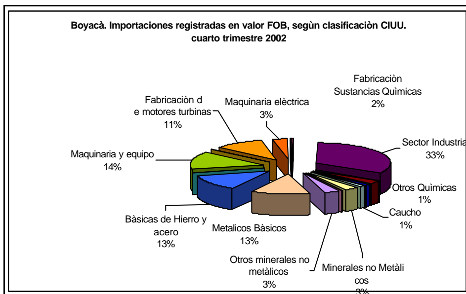
Grafico 5
