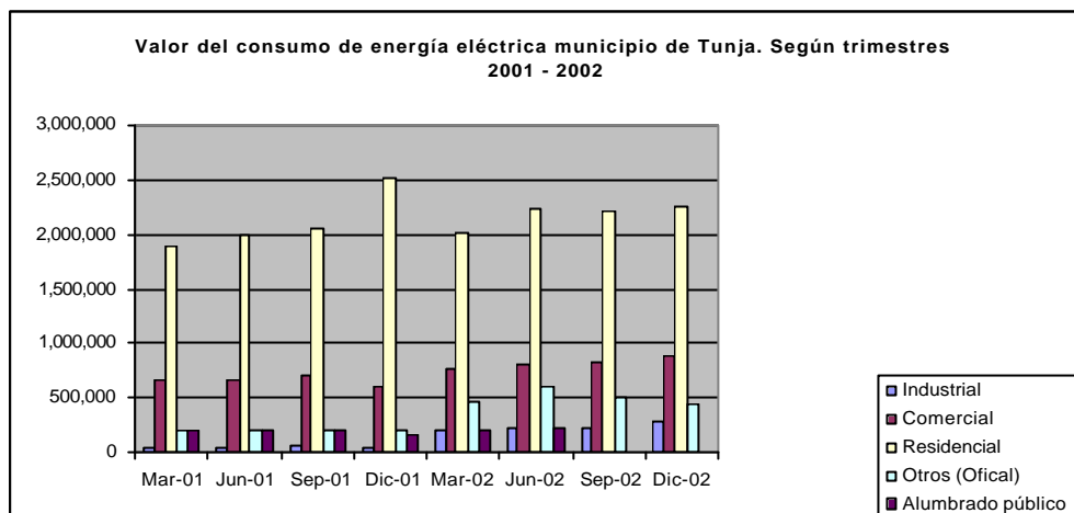
Gráfico 12
