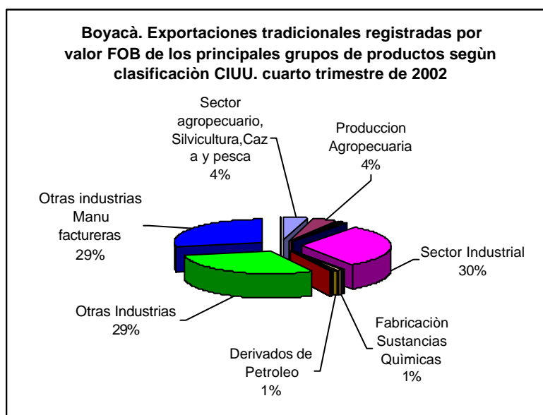
Grafico 3
