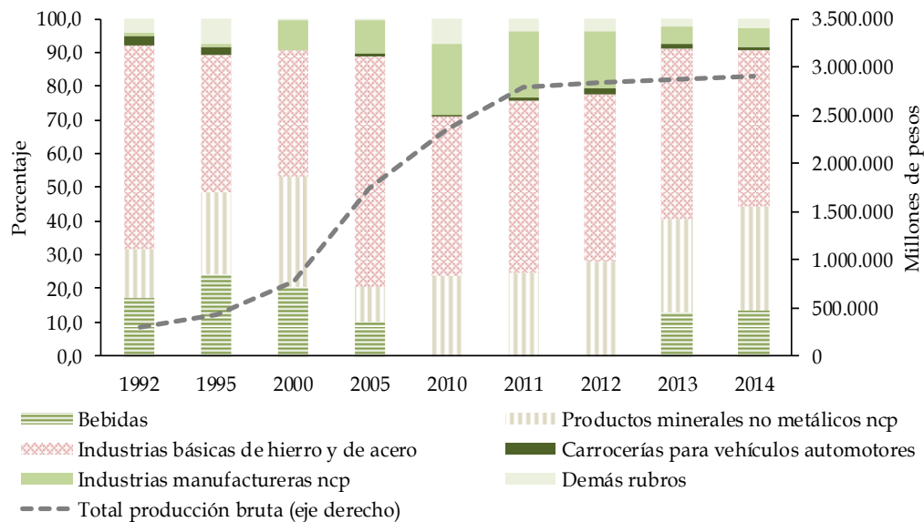
Gráfico 6 Boyacá. Evolución de la producción industrial y su composición, 1992 - 2014 1992-2014
