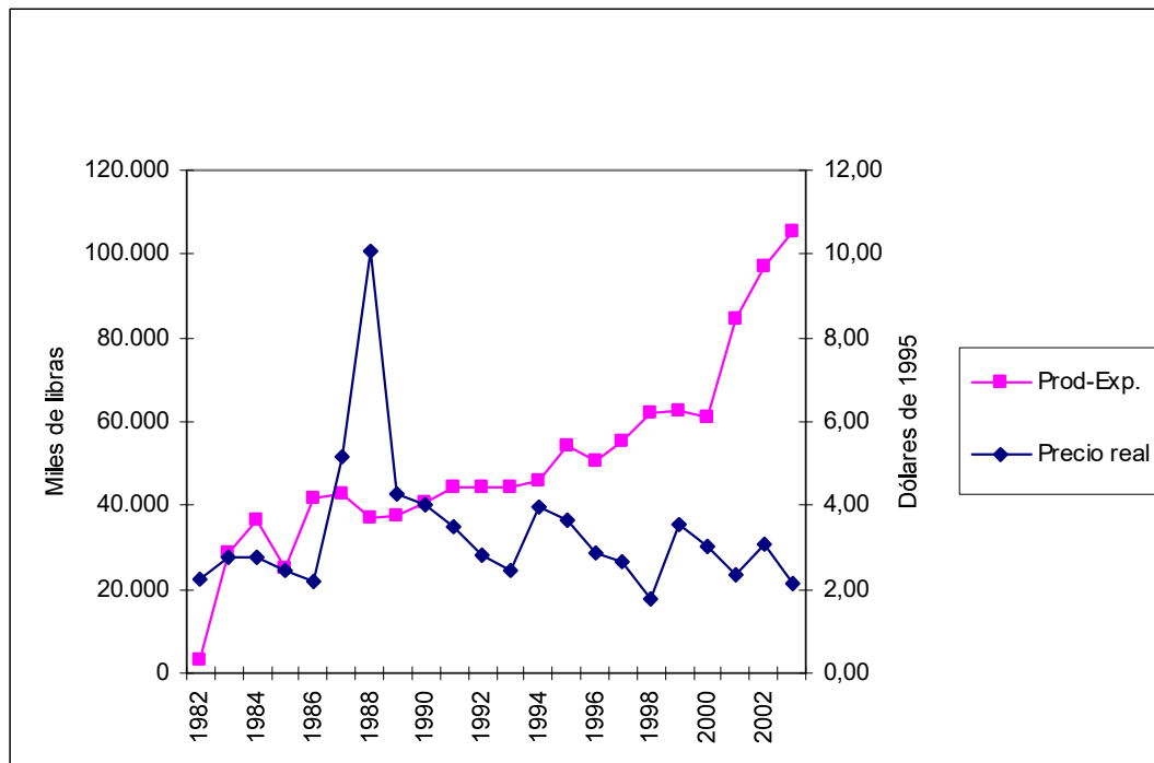
Gráfico 11 Producción-exportación de ferróníquel en el departamento de Córdoba y precio internacional en términos reales, 1982-2003
