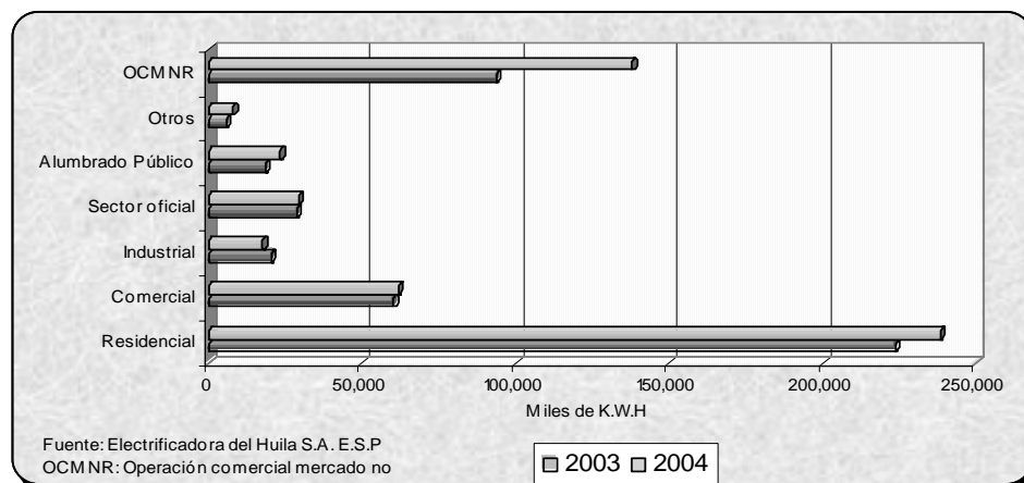
Gráfico 18 Huila. Consumo de energía eléctrica Acumulado años 2003 - 2004
