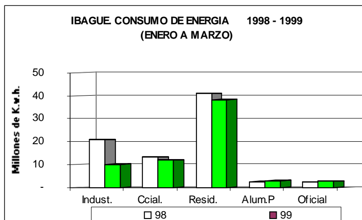
Cuadro No. 12 IBAGUE - CONSUMO DE ENERGIA ELECTRICA (Miles de Kilovatios)
