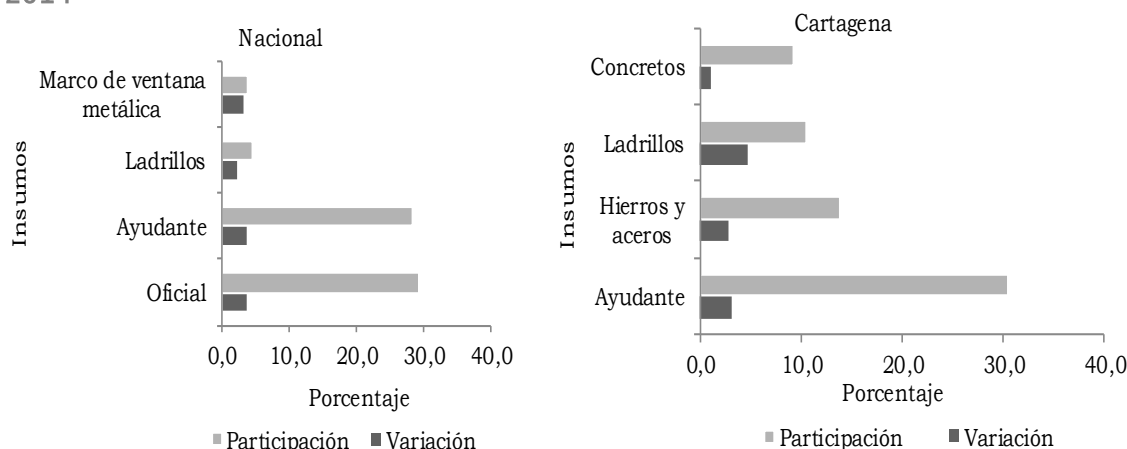
Gráfico 2.8.6.7. Nacional-Cartagena. Variación de insumos básicos con mayor participación 2014
