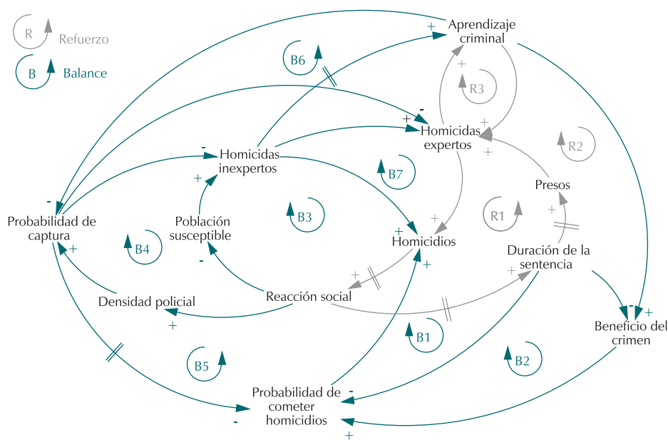
Figura 3 Hipótesis dinámica detallada del modelo del sistema de la carrera criminal y el crimen
