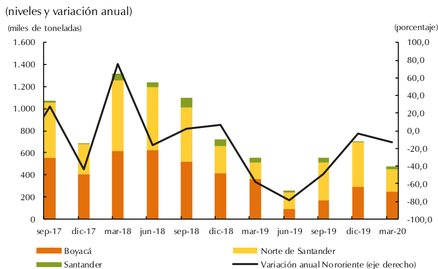
Gráfico 5 Nororiente. Producción de carbón a/
