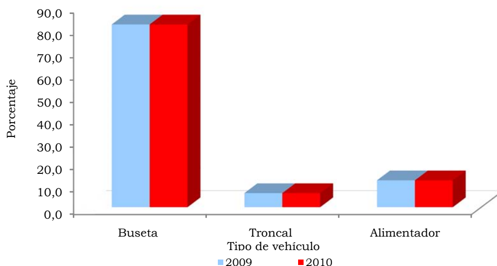
Gráfico 2.8.7.2. Área Metropolitana de Pereira 1 . Distribución de promedio diario de vehículos en servicio 2009-2010
